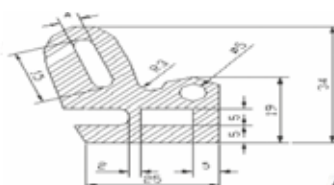
Cód. MA: 03621 Perfil Esponjoso
