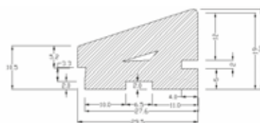
Cód. MA: 03518 Perfil Esponjoso
