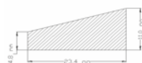
Cód. MA: 03633 Perfil Esponjoso Vedação
