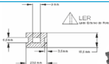
Cód. MA: 03569 Perfil Esponjoso
