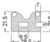
Cód. MA: 03716 Perfil Esponjoso
